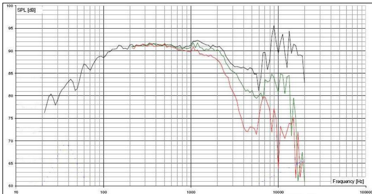
Risposta in frequenza e impedenza del woofer 18W impiegato nella Seconda e Quinta 2011 (misurata su schermo IEC). I break up della membrana del cono in alluminio si trovano oltre i 6000 Hz ben lontane dalla zona di utilizzo. Anche la dispersione è molto regolare con le tre curve ben separate senza sovrapposizioni. Questo risultato è stato ottenuto grazie alla particolare curvatura del cono.
